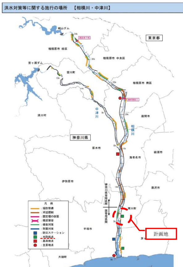
図 2-1 1 水防拠点計画位置図（相模川水系 相模川・中津川河川整備計画）
