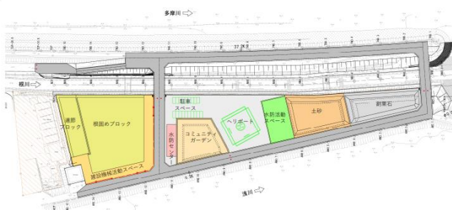
図 2-1 2 水防活動スペースイメージ図（石田地区防災ステーション事例）
