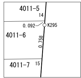
拡大図1 S=1:50
