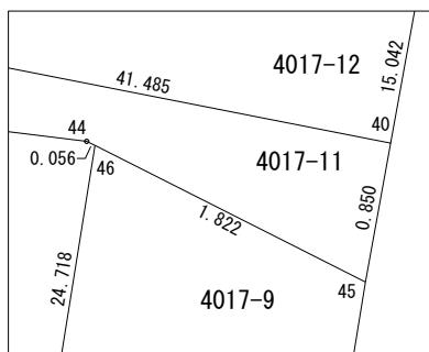
拡大図 S=1:50
