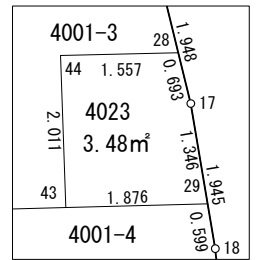
拡大図1 S=1:100
