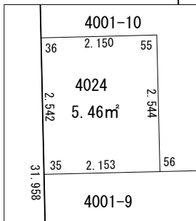
拡大図2 S=1:100
