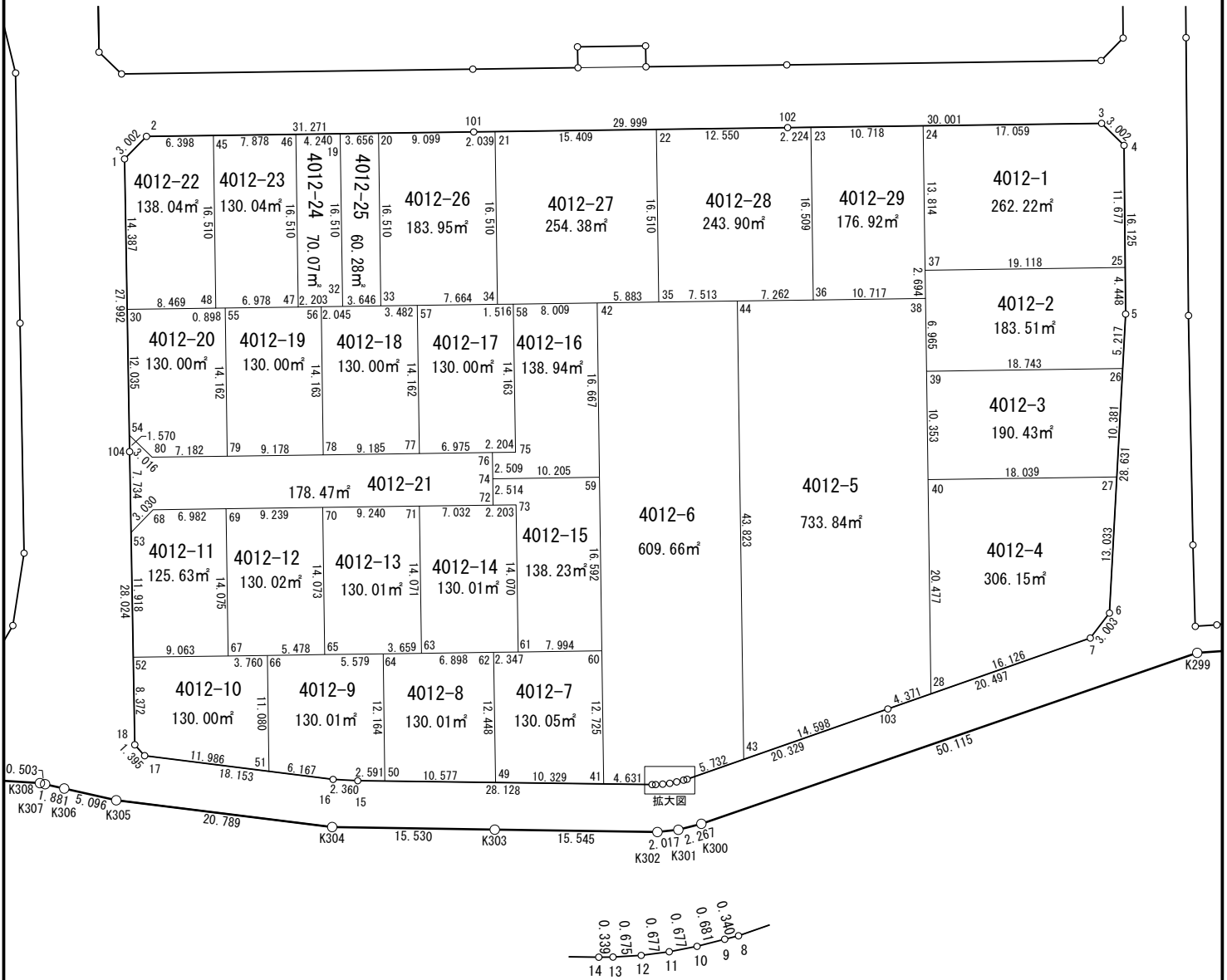
拡大図 S=1:150
