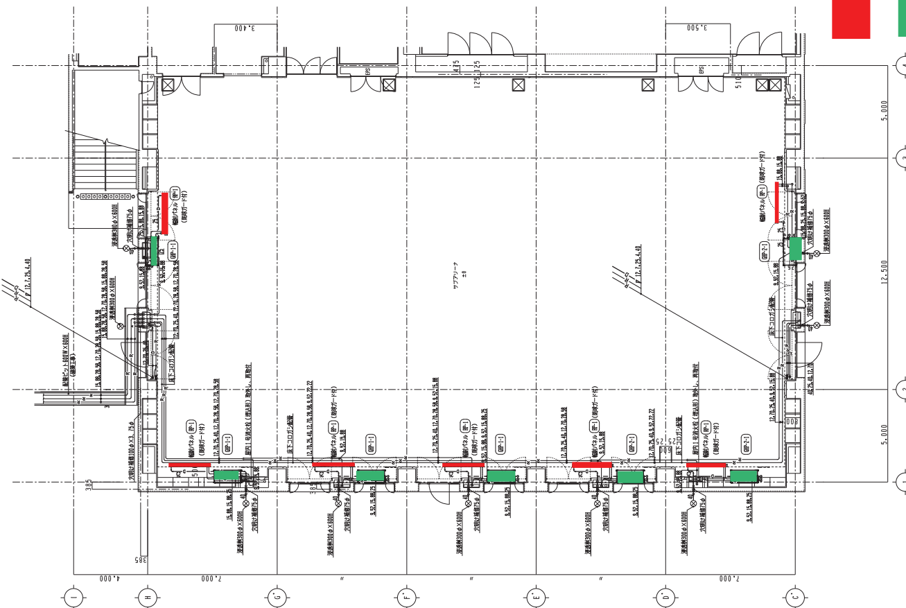
1階サブアリーナ平面詳細図 S=1/100
