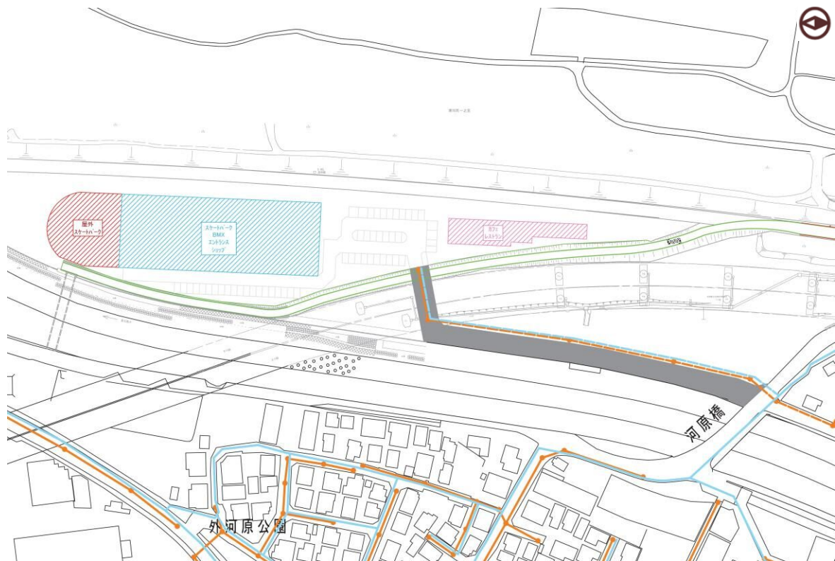
図 2-6 周辺既存道路及び埋設管等の状況図
