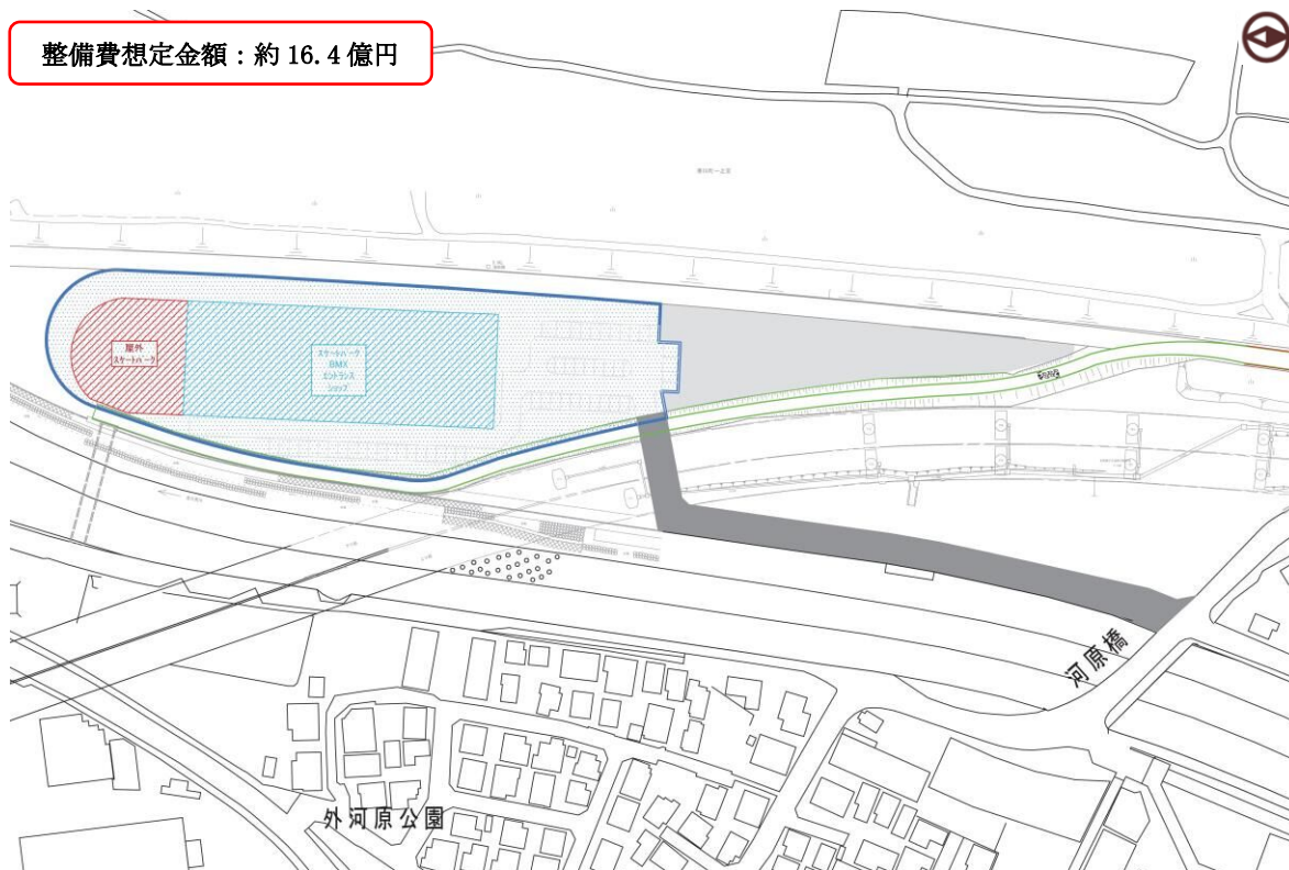
図 2-15 にぎわいの公園機能配置検討図
