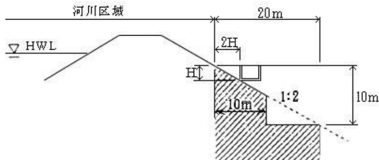
図 2-10 2Hルール概要図
