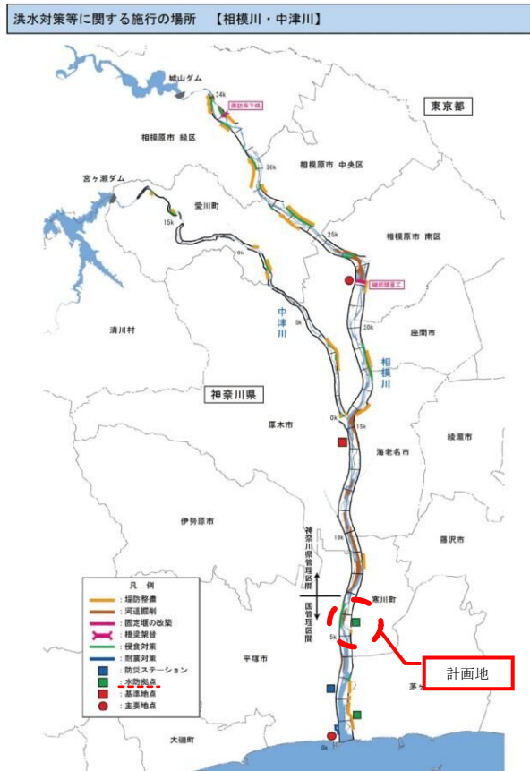
図 2-11 水防拠点計画位置図（相模川水系 相模川・中津川河川整備計画）
