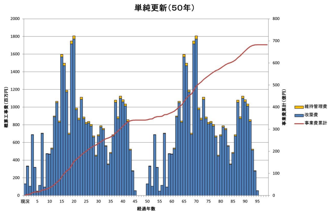
図 11 シナリオ 1 による試算 寒川町下水道長寿命化計画基本構想 より
