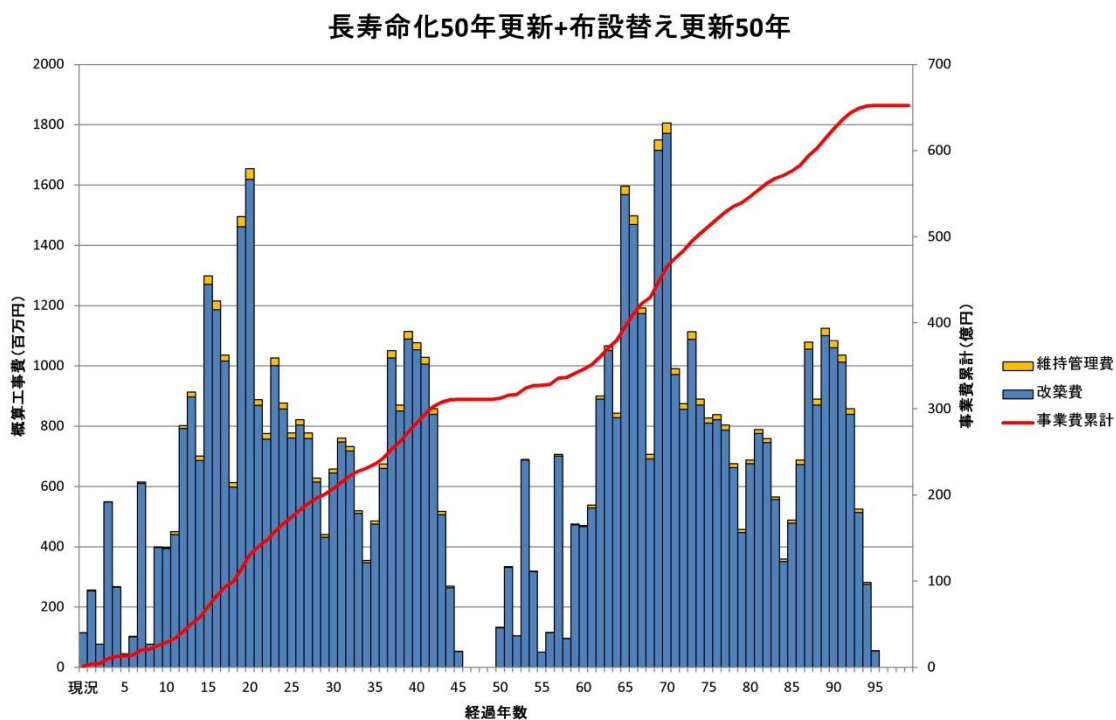
図 12 シナリオ 2 による試算 寒川町下水道長寿命化計画基本構想 より
