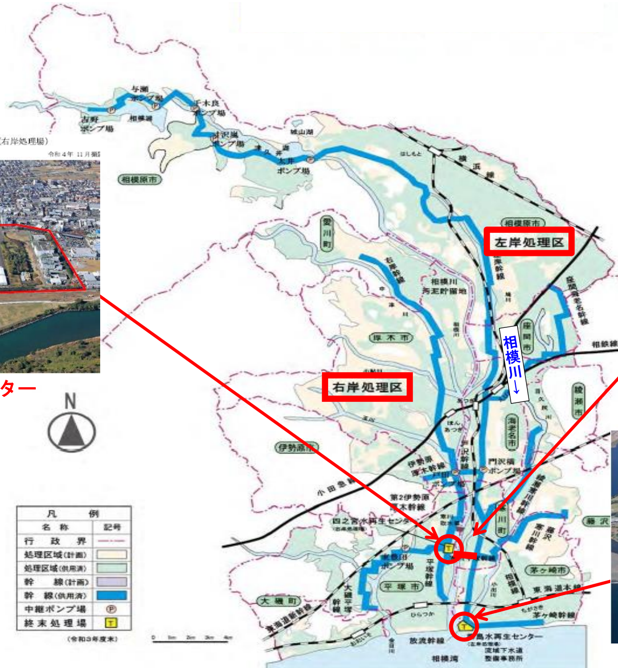
相模川流域下水道 柳島水再生センター（左岸処理場）
