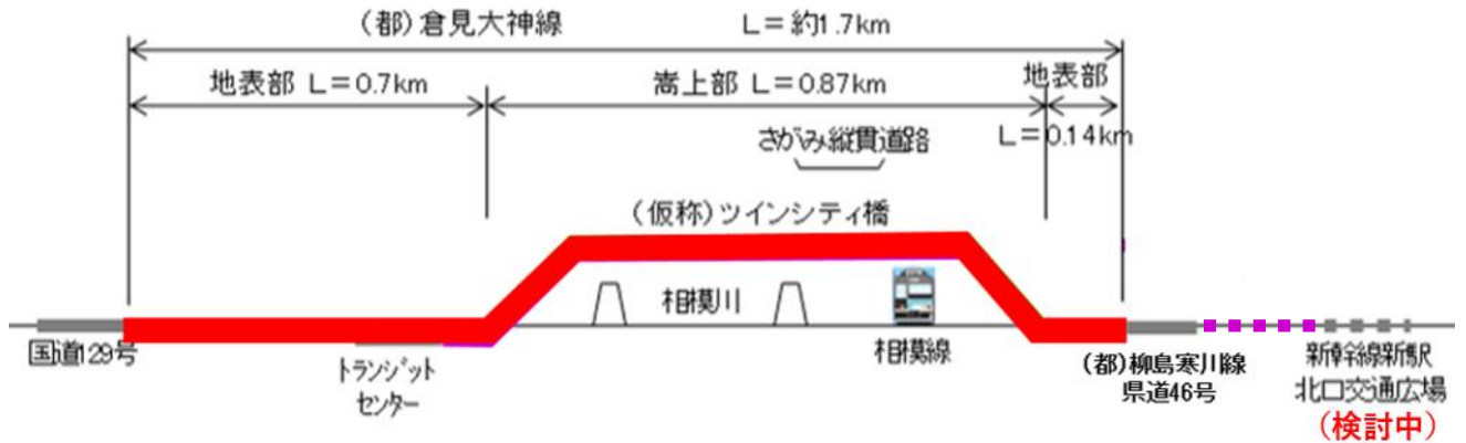
縦断図
