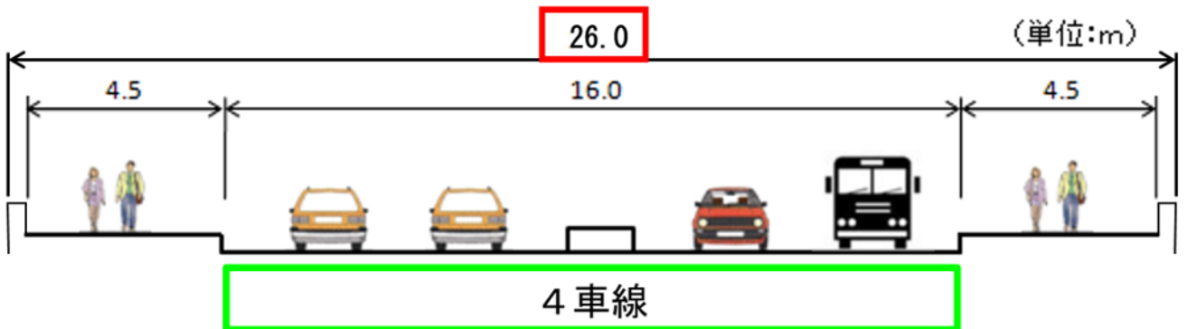
標準横断図 (橋梁部)
