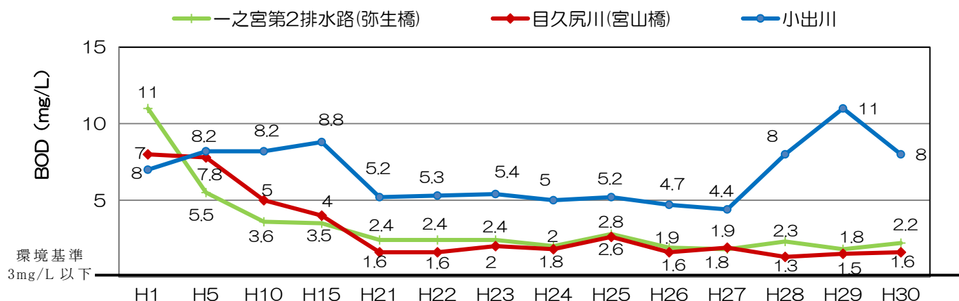
BODの経年変化（75%値）
