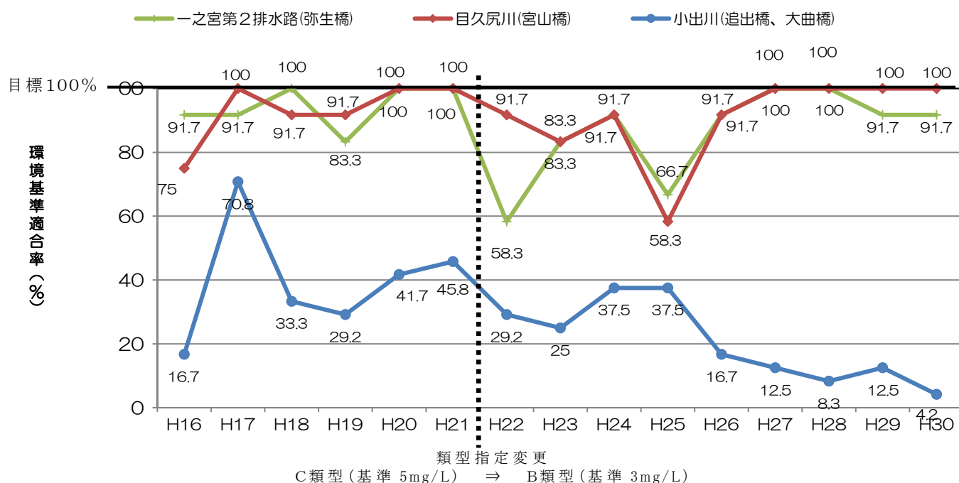
BOD環境基準適合率の推移
