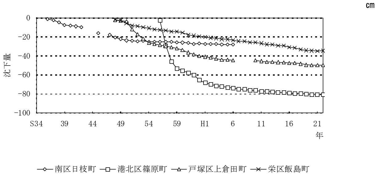
図4-2 主要水準点の累計沈下量 横浜地域 (2)
