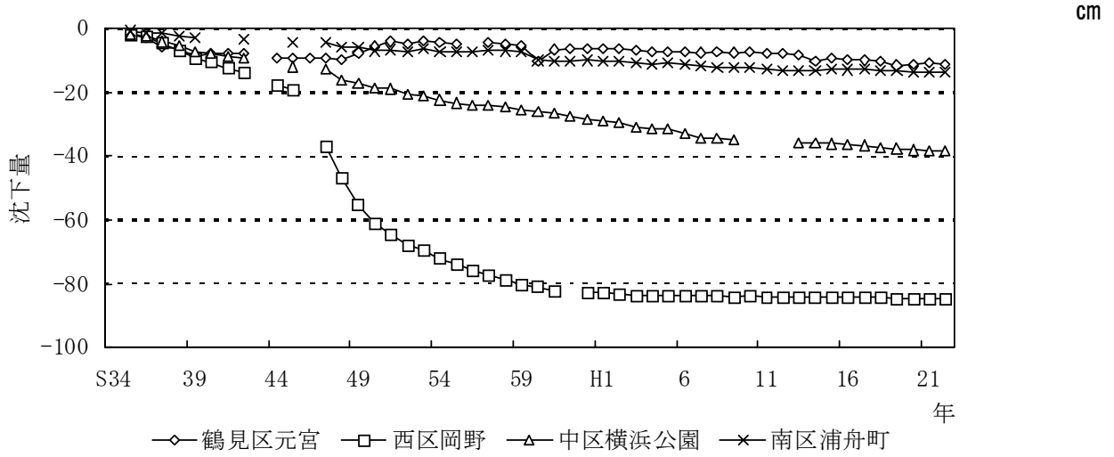
図4-1 主要水準点の累計沈下量 横浜地域 (1)
