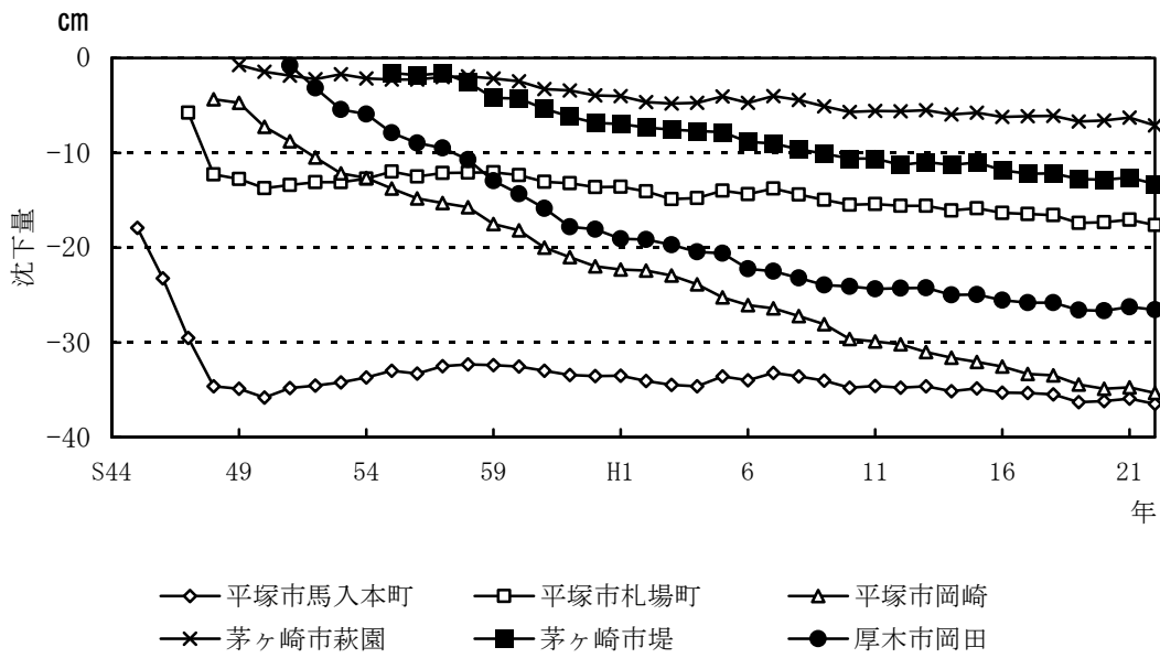
図6-1 主要水準点の累計沈下量 県央・湘南地域 (1)
