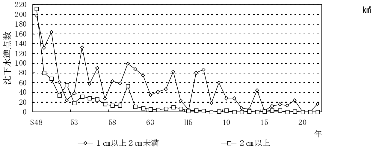
図3-1 地盤沈下状況の経年変化（沈下水準点数）
