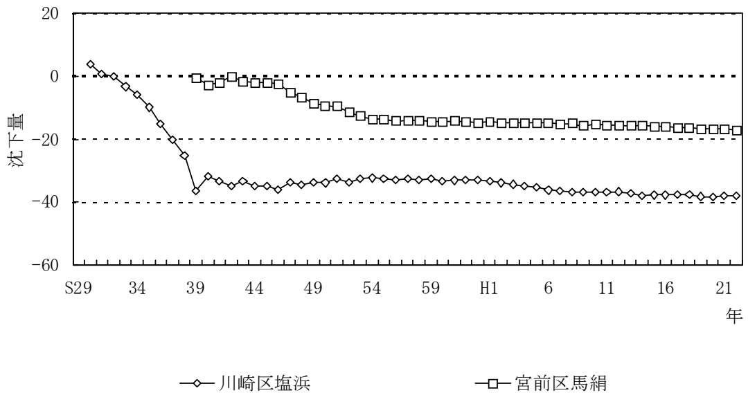
図5-2 主要水準点の累計沈下量 川崎地域 (2)
