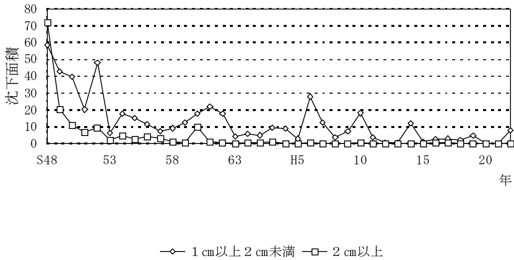
図3-2 地盤沈下状況の経年変化（沈下面積）
